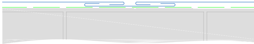
1. - Roofinox - Stossverbinder unterlegt (Abdeckung, mit Querneigung \geq 3^\circ oder Breite \geq 0,50 m)
