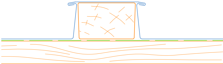
Deutsche Leistendeckung Höhe 40 mm, Dachneigung \geq 7^\circ Roofinox Zinn-matt: immer mit Falzgel, unabhängig von der Dachneigung
