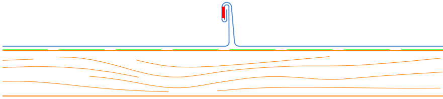
Doppelstehfalz, Höhe 25 mm mit Roofinox Falzgel Dachneigung \geq 3^\circ
