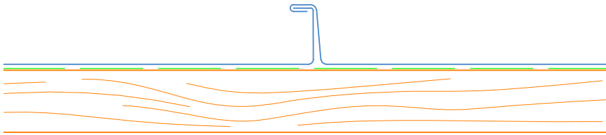
Winkelfalz, Höhe 25 mm Dachneigung \geq 25^\circ Roofinox Zinn-matt: immer mit Falzgel, unabhängig von der Dachneigung
