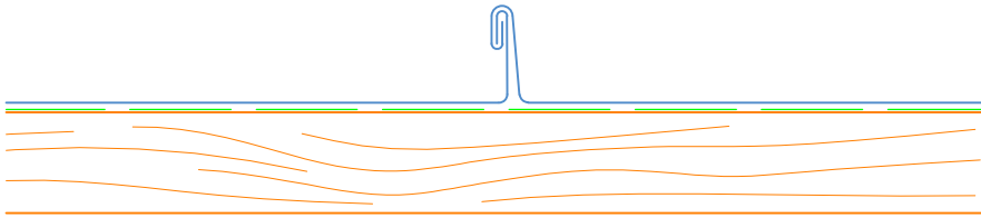
Doppelstehfalz, Höhe 25 mm Dachneigung \geq 7^\circ Roofinox Zinn-matt: immer mit Falzgel, unabhängig von der Dachneigung
