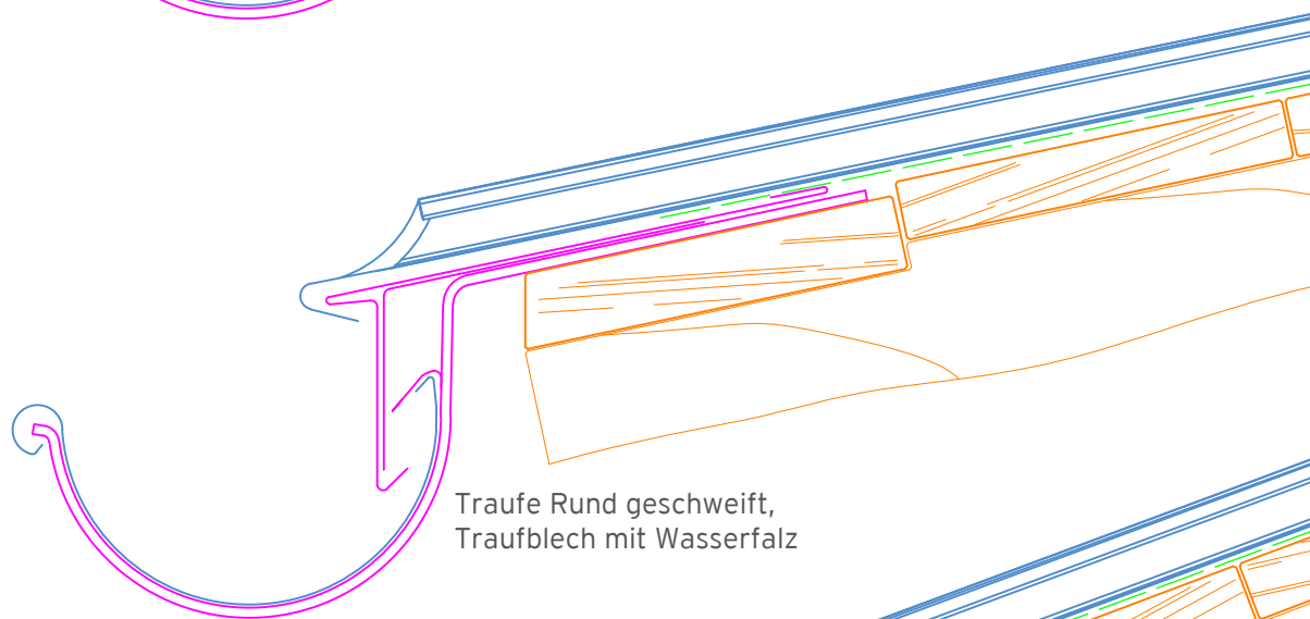
Traufe Schwäbisch, Traufblech mit Wasserfalz
