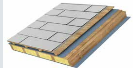
DACHAUFBAU
